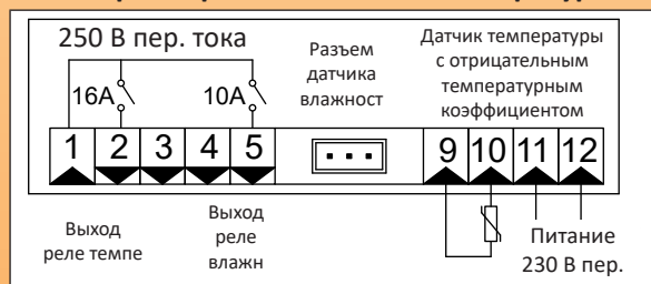
Схема электрических соединений контроллера влажности и температуры
