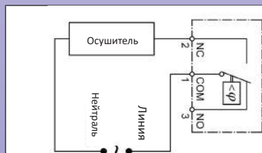
Система осушения воздуха
